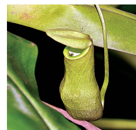
Nepenthes
