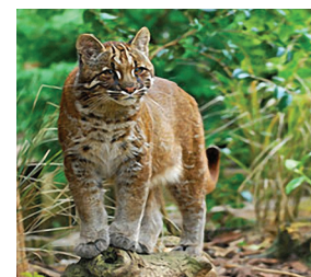
Wild cat
