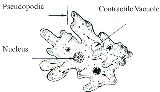
Fig-9(b) Amoeba
