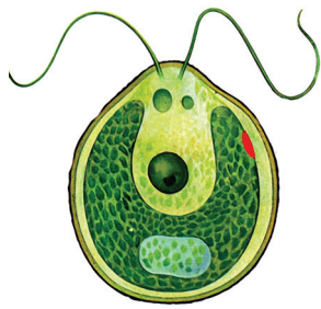
Fig-9(a) Chlamydomonas
