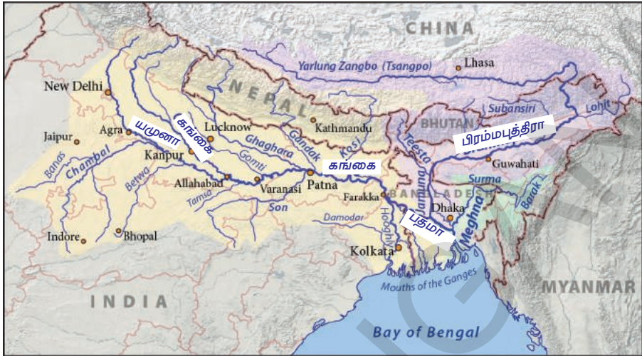
படம் 5.2 கங்கைநதி பிரம்மபுத்திராவடன் இணைதல்
