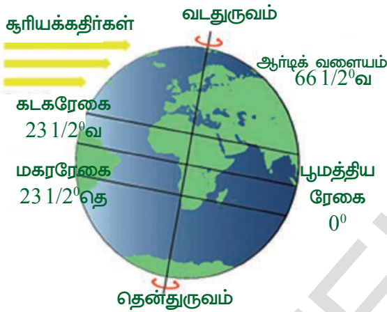
படம் 4.5 : காலநிலை மீது அட்சரேகையின் தாக்கம்
