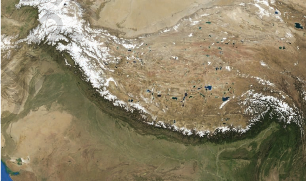
படம் 1.2 : செயற்கைக்கோளிலிருந்து படமாக்கப்பட்ட இமயமலை, வடக்குத் சமவெளி மற்றும் தார்பாலைவனம்.
