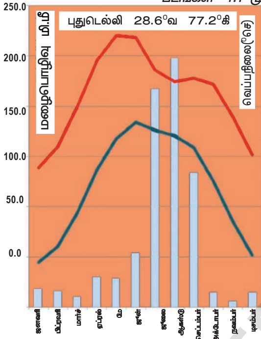
படங்கள் 4.1 முதல் 4.4 காலநிலை வரைபடங்கள்
