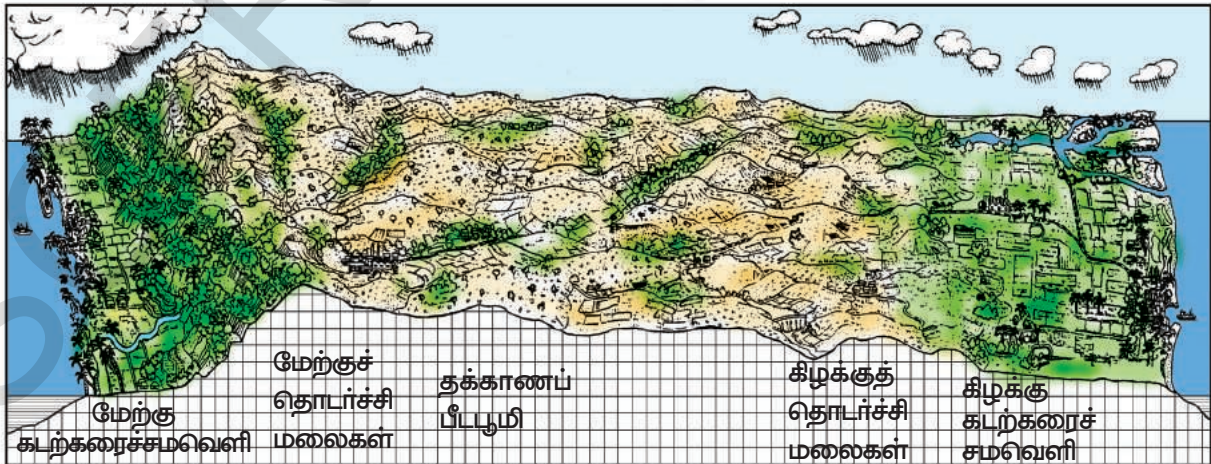
படம் 1.9 : தீபகற்ப பீடபூமியின் விளக்க வரைபடம்
