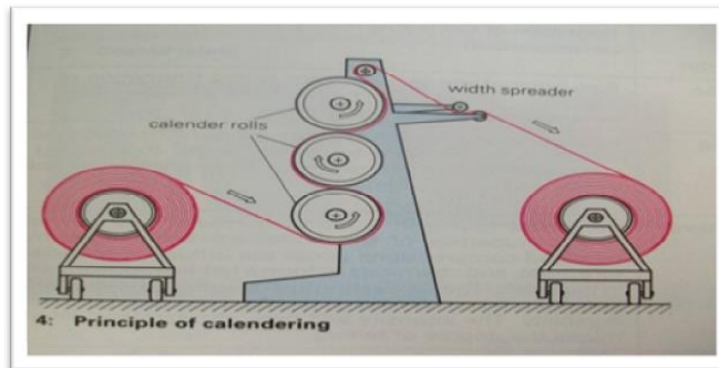
ਚਿੱਤਰ 2.27 : ਕੈਲੇਂਡਰਿੰਗ
