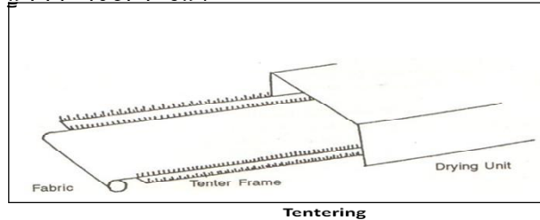
ਚਿੱਤਰ 2.28 : ਟੈਂਟਰਿੰਗ
