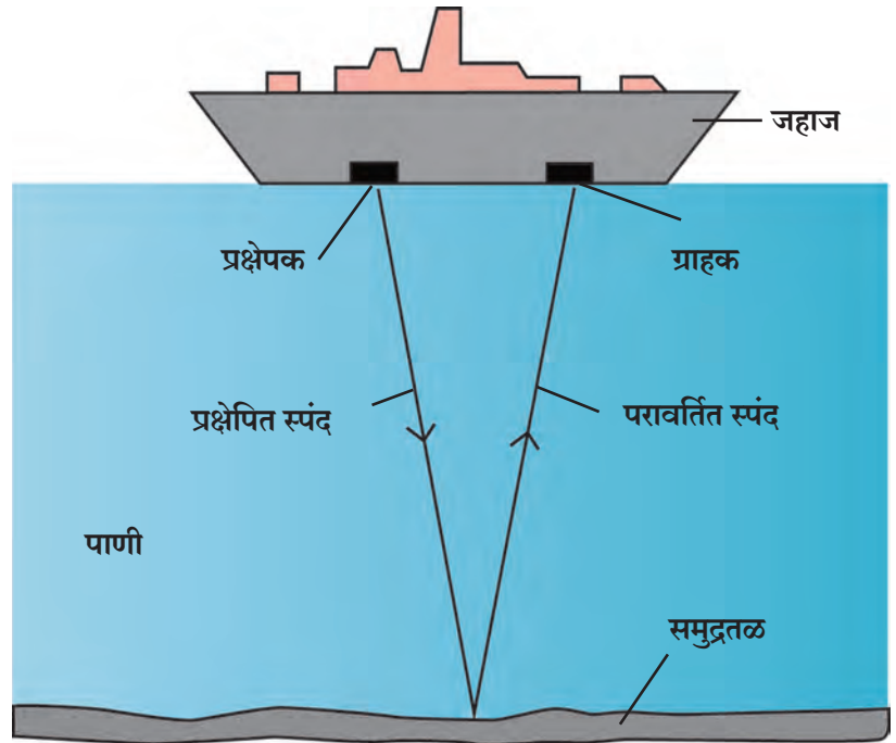
12.4 सोनार पद्धत
