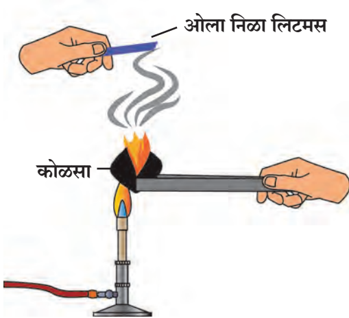
13.9 कार्बनची ऑक्सिजनबरोबर अभिक्रिया
