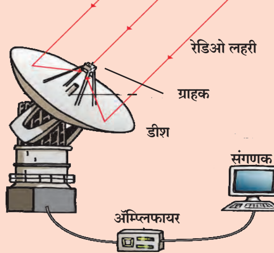
18.4 (अ) रेडिओ दुर्बिणीची रचना (ब) रेडिओ दुर्बिणीचे छायाचित्र
