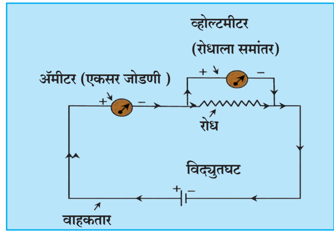
3.5 विद्युत परिपथ
