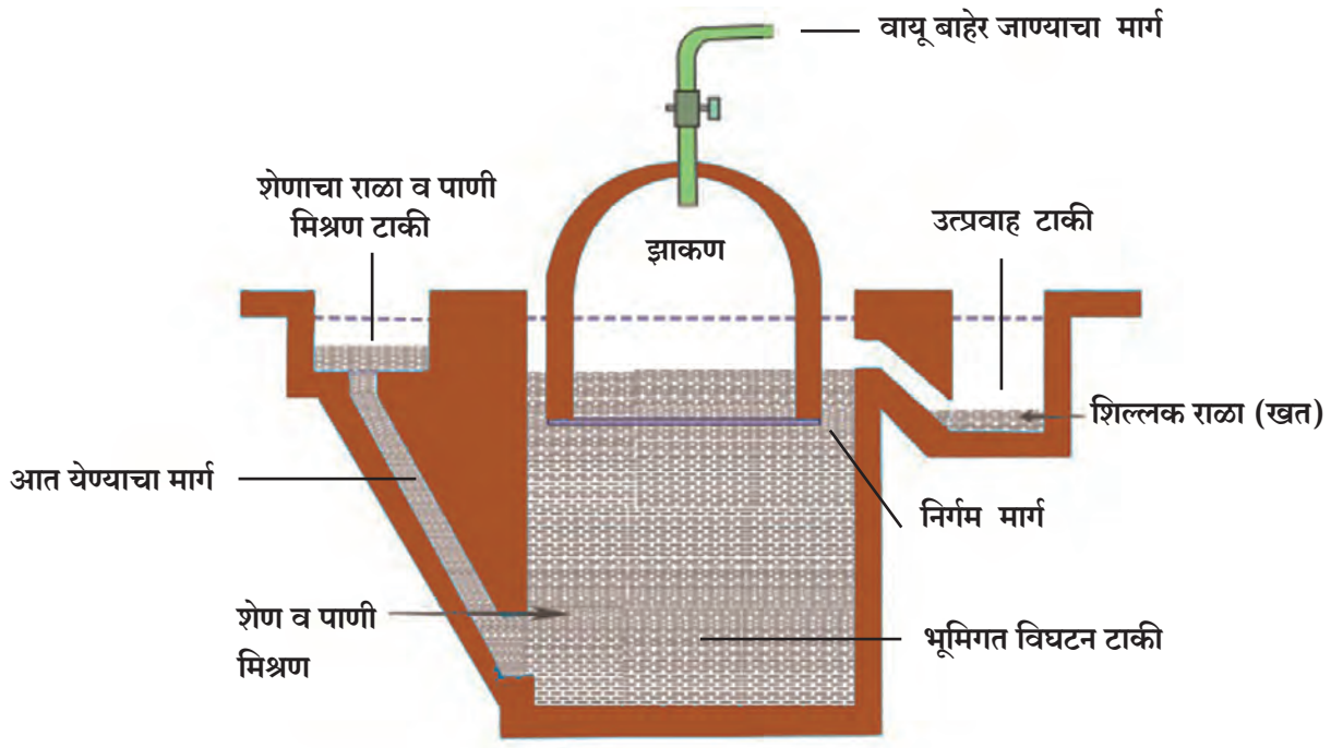
13.13 बायोगॅस संयंत्र
