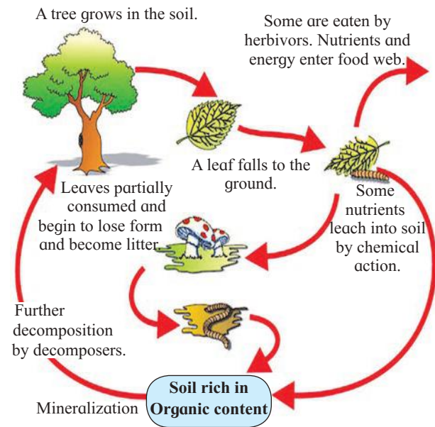
Fig. 14.3 : Decomposition cycle
