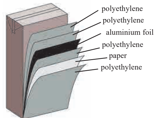
Fig. 14.20 : Tetra brik aseptic package
