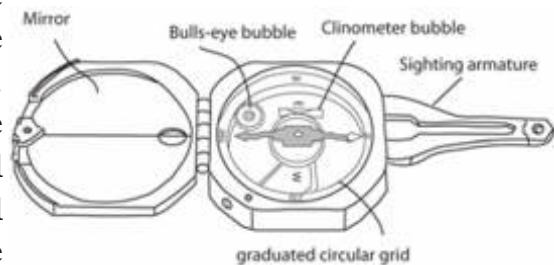
Fig. 4.7: Brunton Compass
