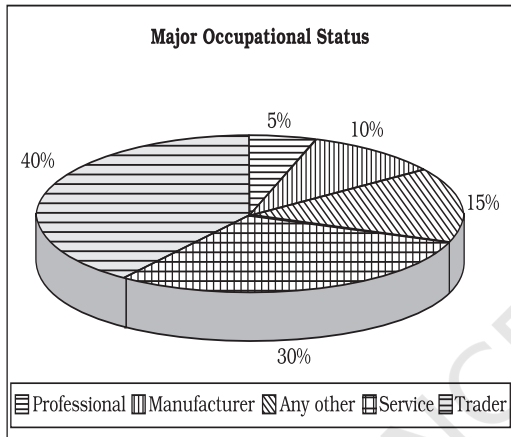
Fig. 9.4: Pie diagram
