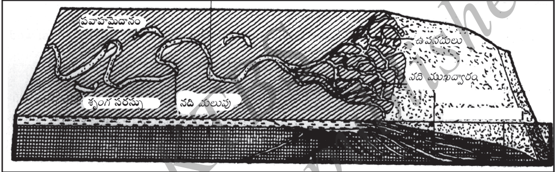
నది ప్రవాహాల వలన ఏర్పడిన భూ స్వరూపాలు
