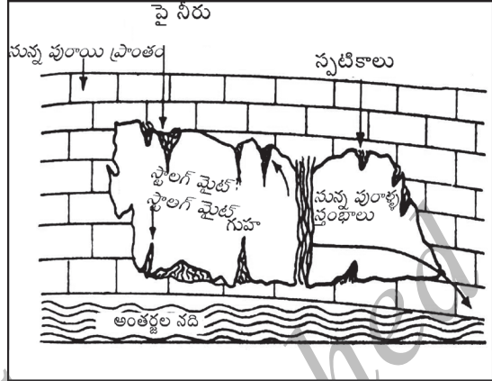
భూగర్భ జలం కార్యం
