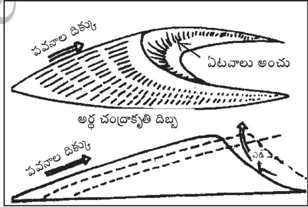
అర్ధచంద్ర ఆకారం గల ఇసుక దిన్నె-భార్గనులు
