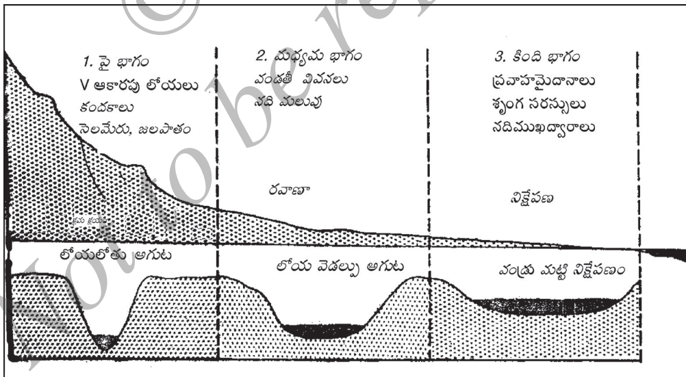
నదీ ప్రవాహాల వివిధ మట్ట ములు, దానికి సంబంధించిన భూ స్వరూపాలు.
