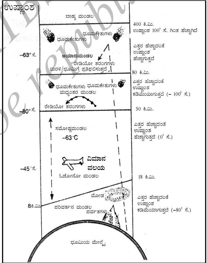
ವಾಯುಮಂಡಲ ಸ್ತರಗಳು
