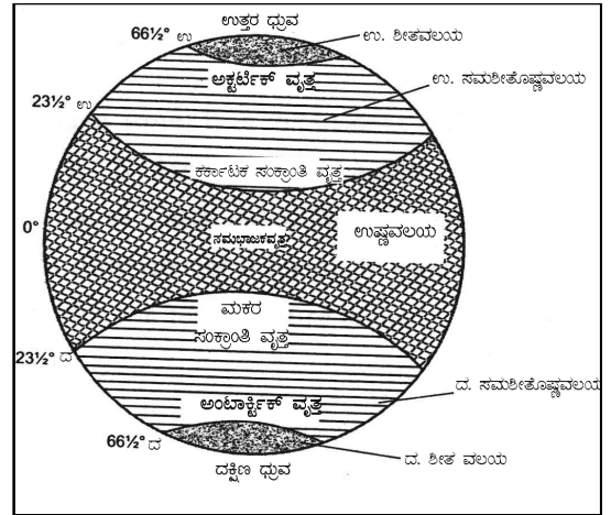
ಉಷ್ಣಾಂಶ ವಲಯಗಳು
