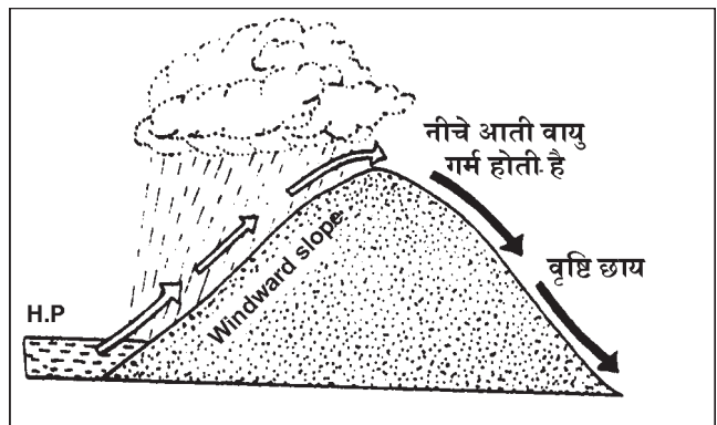
पर्वतीय वर्षा
