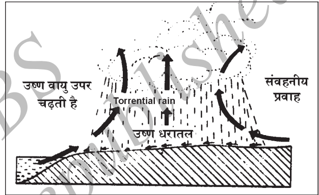
संवहनीय वर्षा
