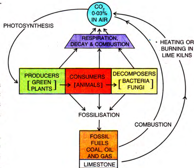
Fig. 6.10 : Carbon cycle
